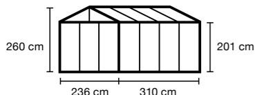
M23 - 7,3 m 2 - 16,83 m 3
