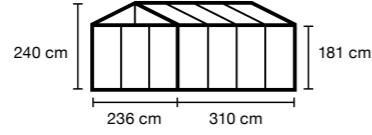
S23 - 7,3 m 2 - 15,37 m 3
