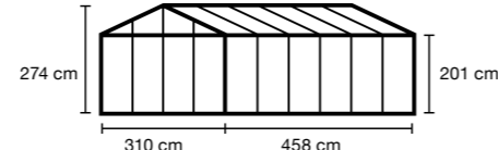
M34 - 14,2 m 2 - 33,61 m 3
