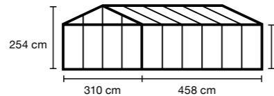
S34 - 14,2 m 2 - 30,78 m 3
