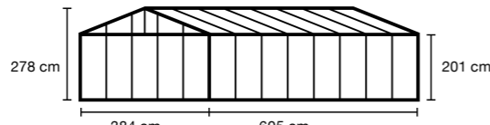
M46 - 23,3 m 2 - 55,51 m 3
