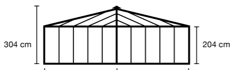
P44 - 14,7 m 2 - 37,35 m 3
