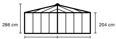
P33 - 9,6 m 2 - 23,52 m 3
