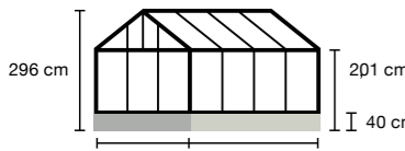
J23 - 7,3 m 2 - 18,15 m 3
