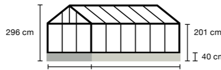
J25 - 10,8 m 2 - 26,79 m 3
